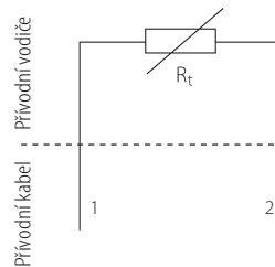
Dvouvodičové
