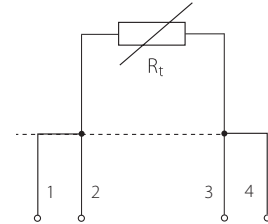
Čtyřvodičové
