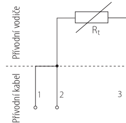
Třívodičové
